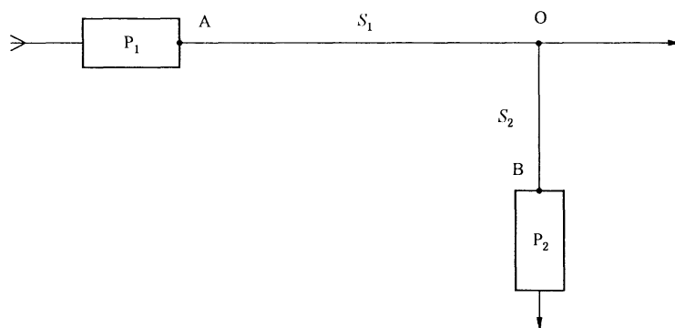
图 C.1 过负荷保护电器( P_2 )不在分支回路(B)的起点(见 433.2.2 a))
