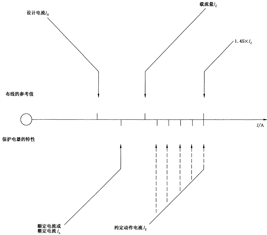
图 B.1 433.1 的条件(1)和条件(2)的说明
